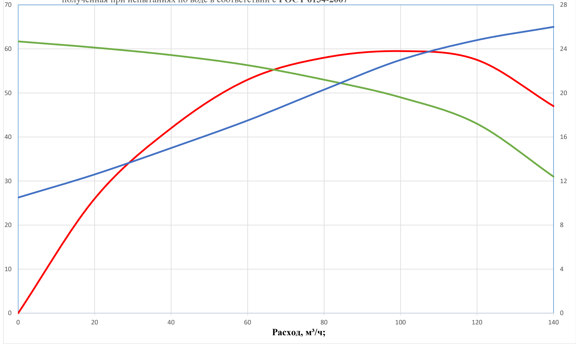
Напор Напорно-энергетическая характеристика — КПД, (%) — Н, (м) — N, (кВт) ОНЦс (ХМс) 100/50К5-30,0/2 с закрытым рабочим колесом Ø210мм. полученная при испытаниях по воде в соответствии с ГОСТ 6134-2007 Мощность, кВт;
